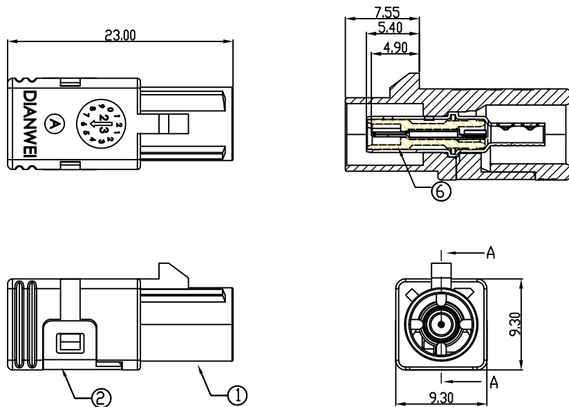
组装线缆后的连接器尺寸
