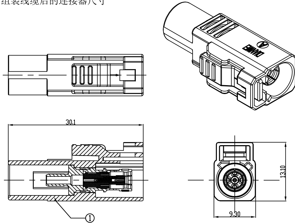
组装线缆后的连接器尺寸
